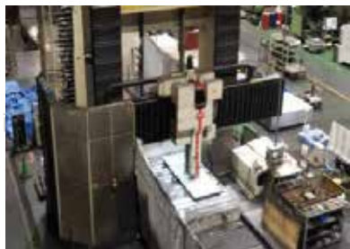
大型五面加工機 (新日本工機 HF-6M)
